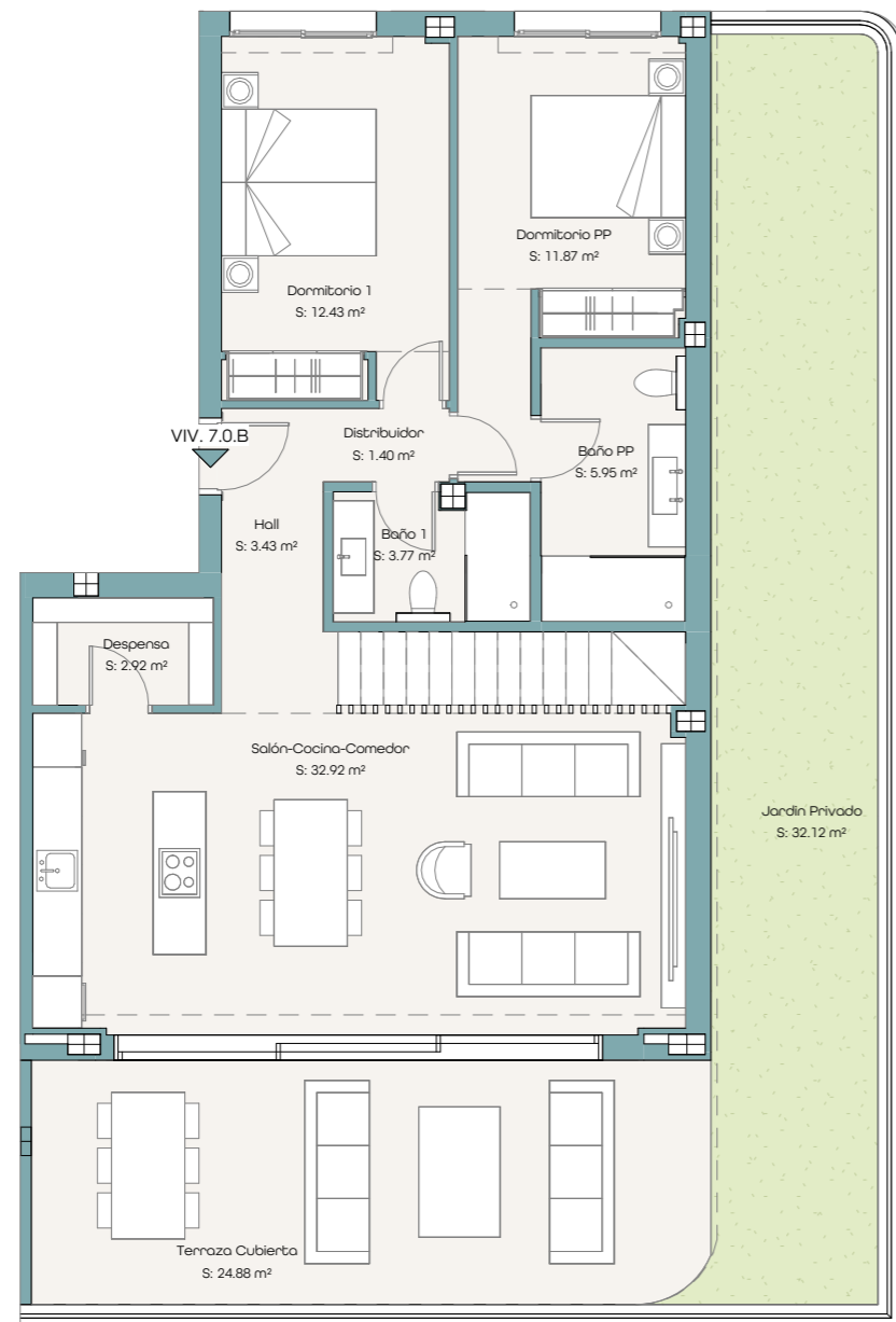
PLANTA BAJA
