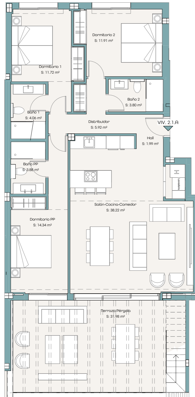
PLANTA PRIMERA
