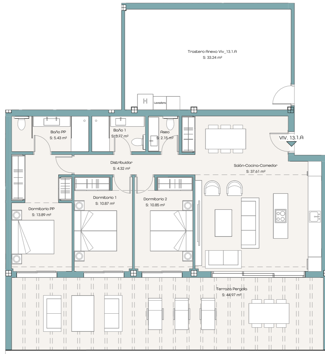
PLANTA PRIMERA
