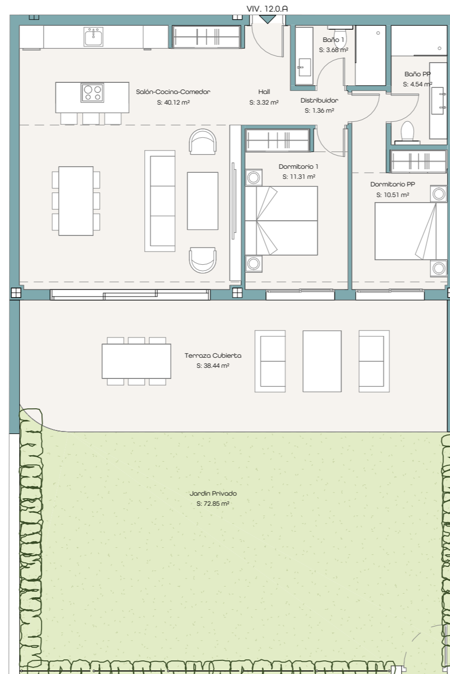
PLANTA BAJA
