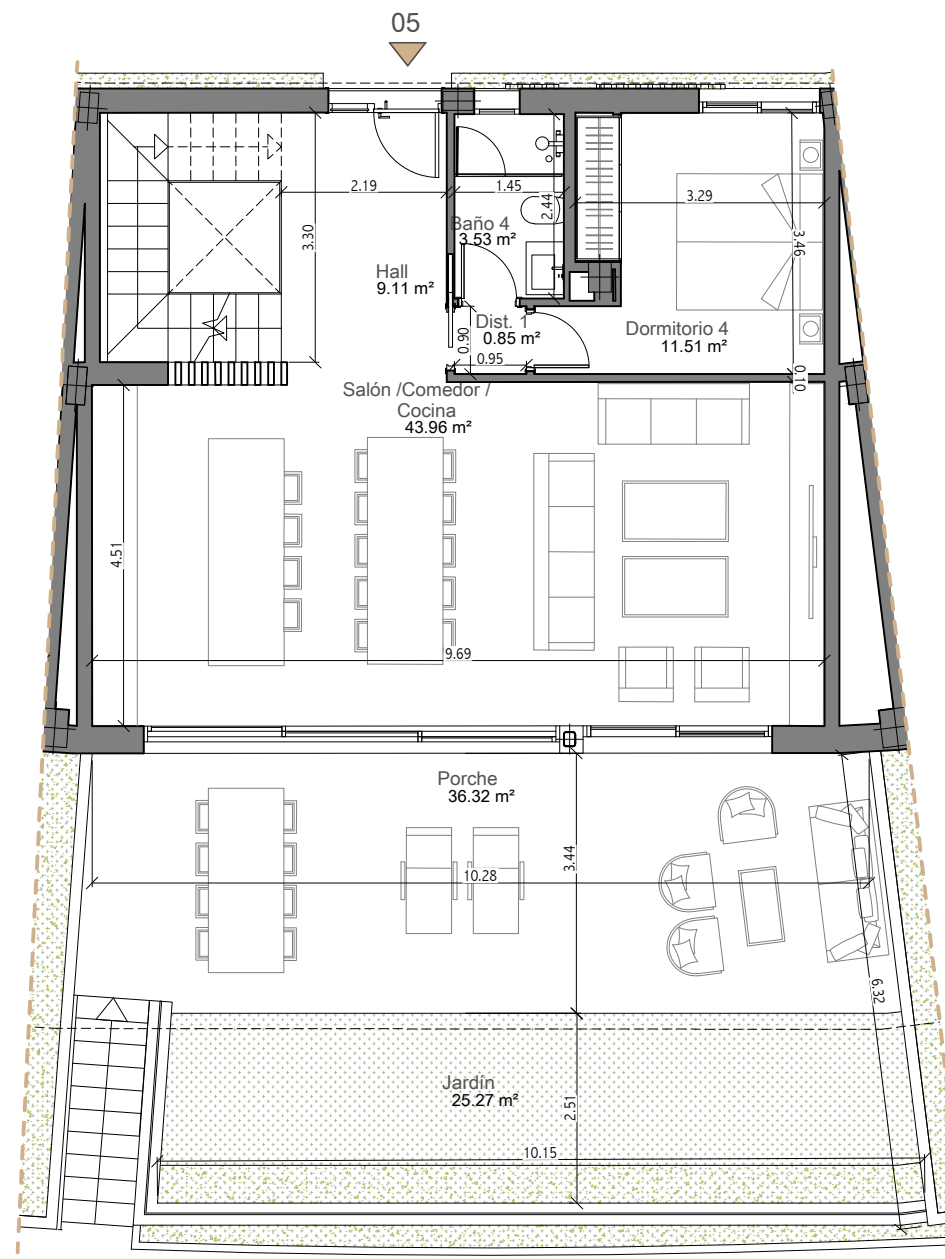
Planta Baja
