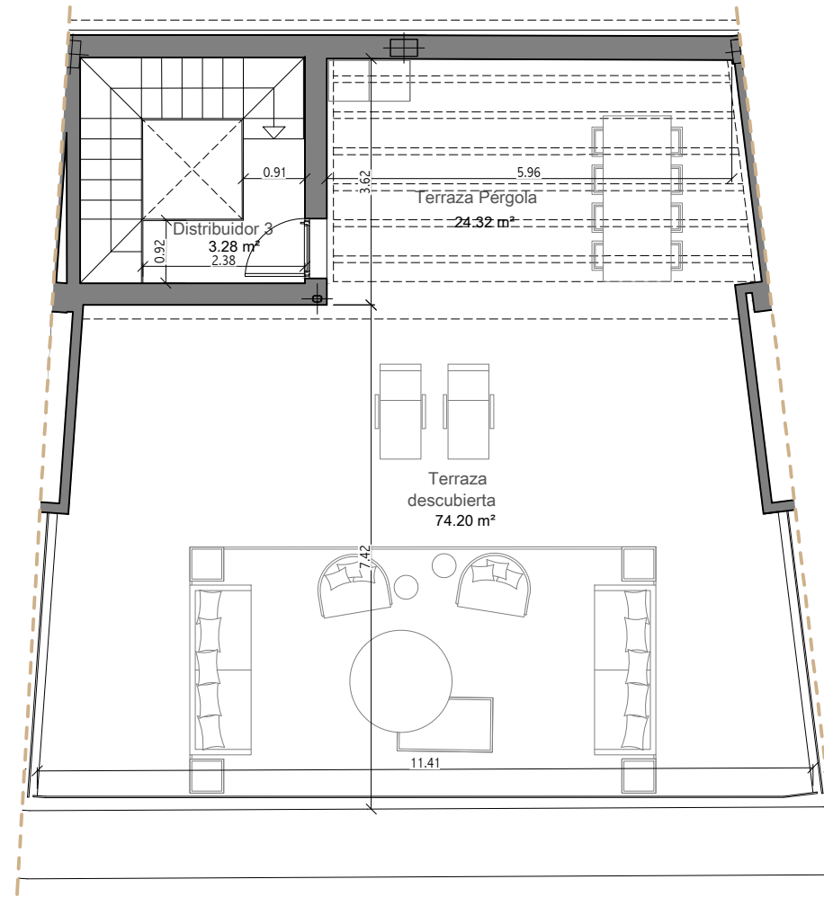
Planta Solarium
