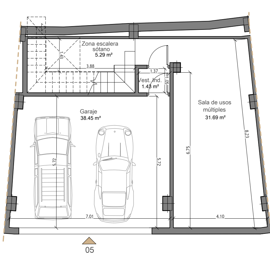
Planta Sótano
