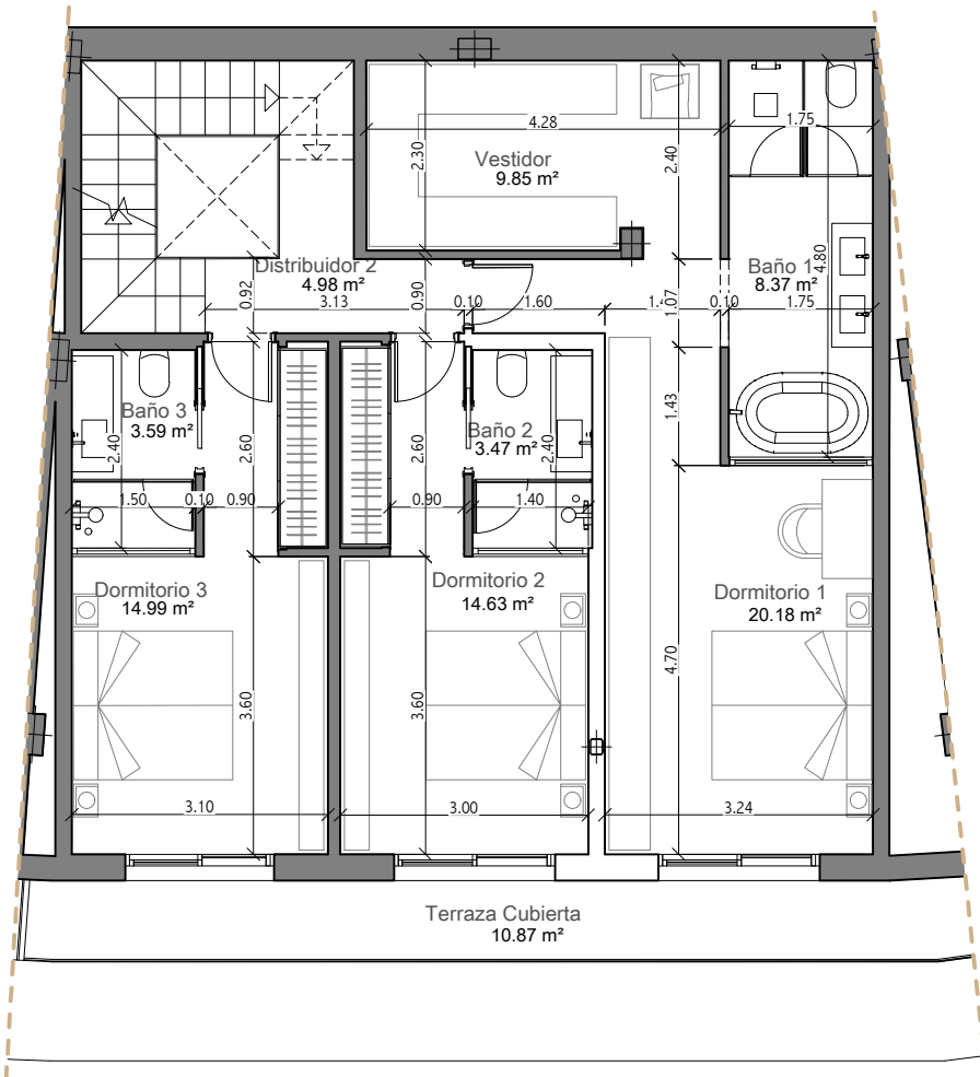
Planta Primera
